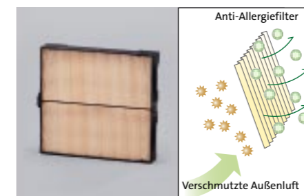
93 Anti-Allergiefilter G3010SA110 ★W Catechin, ein Antiallergikum aus der grünen Tee-pflanze ist dem Filter zugesetzt, um die Filterleistung zu erhöhen. Um die Wirkung zu erhalten, sollte der Filter jährlich oder alle 12.000 km gewechselt werden.
