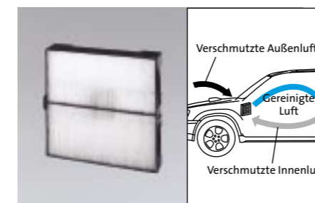
92 Innenluftfilter G3010SA100 ★W Verringert das Eindringen von Staub und Pollen in den Innenraum. Um die Wirkung zu erhalten, sollte der Filter jährlich oder alle 12.000 km gewechselt werden.
