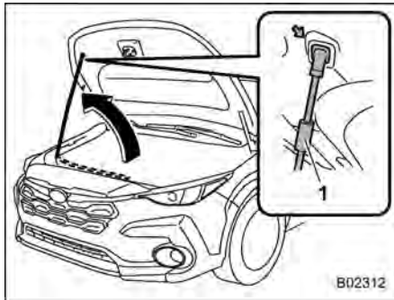
1 Griff
