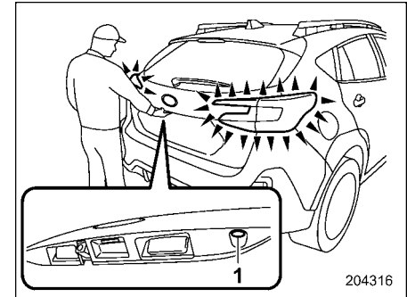
1 Heckklappenverriegelungstaste
