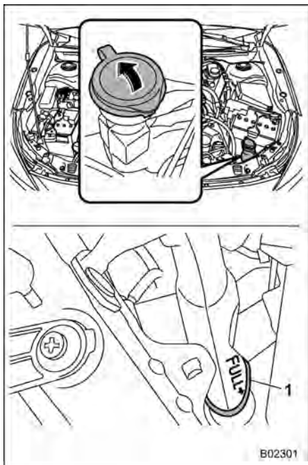
1 "FULL"-Markierung
